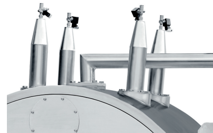
Функция охлаждения: гидравлическая крышка с рожками для подачи снега. Альтернативно: подача CO2 / LN2 через форсунки в днище воронки
